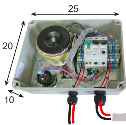
Alimentation 230 V
