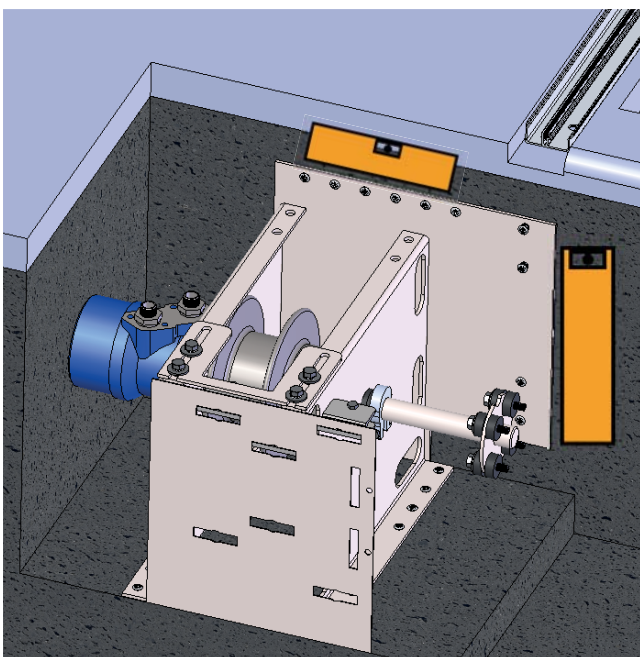
Mise de niveau
