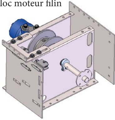
Bloc moteur filin
